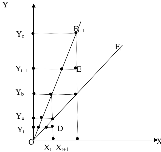
نمودار ۳. تفکیک تغییرات بهره‌وری کل (شاخص مال‌م کوئیس)
